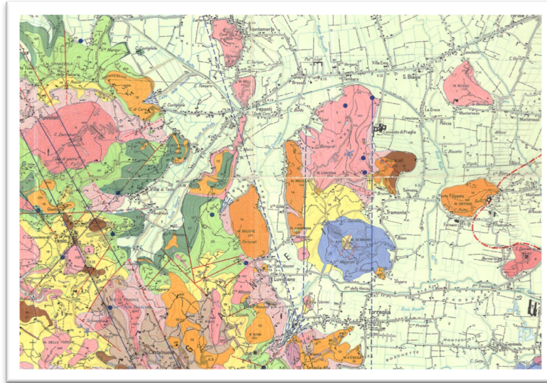
CARTA GEOLOGICA DEI COLLI EUGANEI
